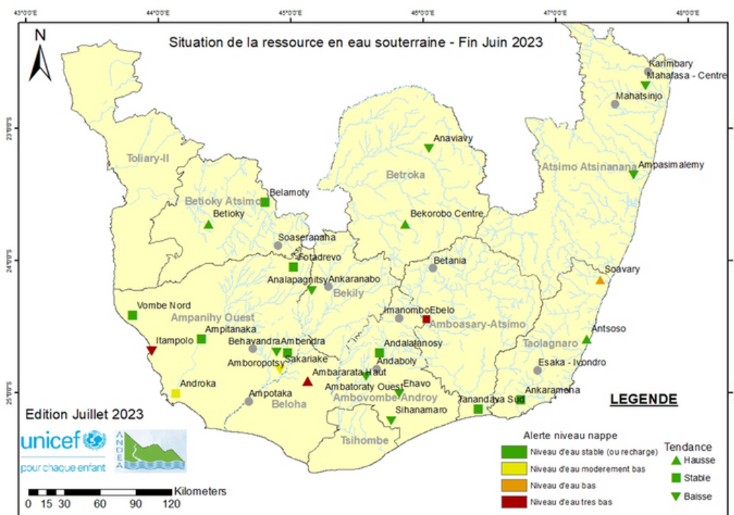
Fig. 2 Etat des niveaux d'eaux souterraines fin Juin 2023
