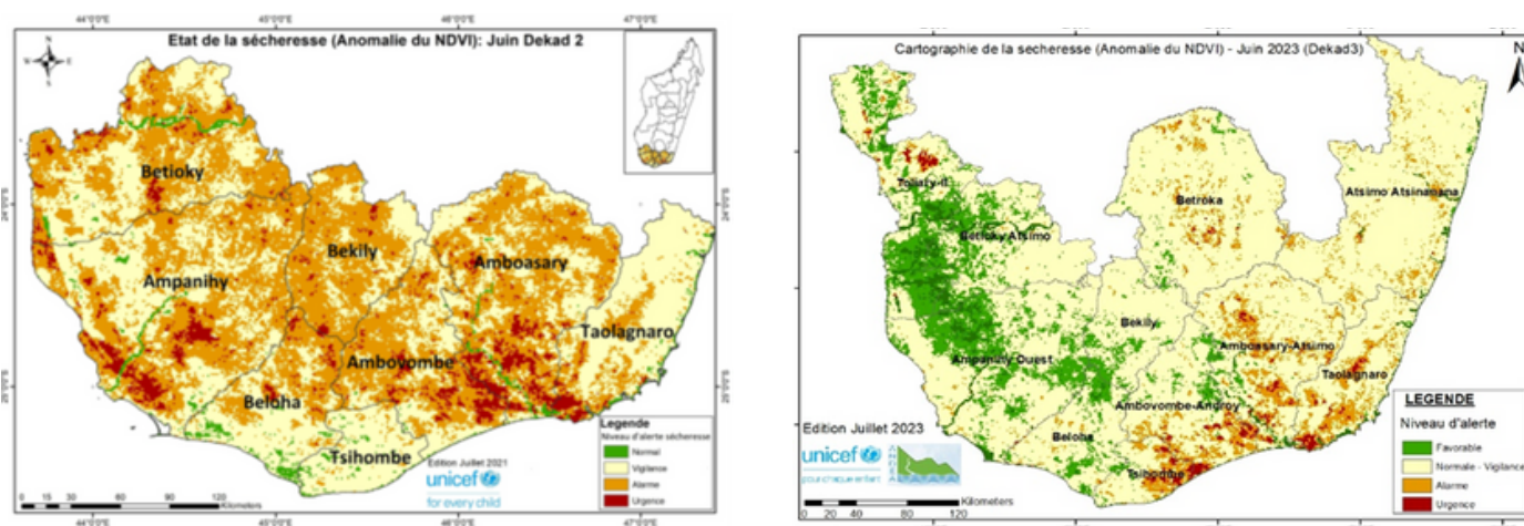
Fig. 3. Comparaison Précipitation/ NDVI 2021/2023 situation Juin 2023
