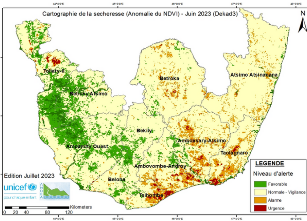
Fig. 1 : Etat de la sécheresse (anomalie NDVI) Juin Décade 3
